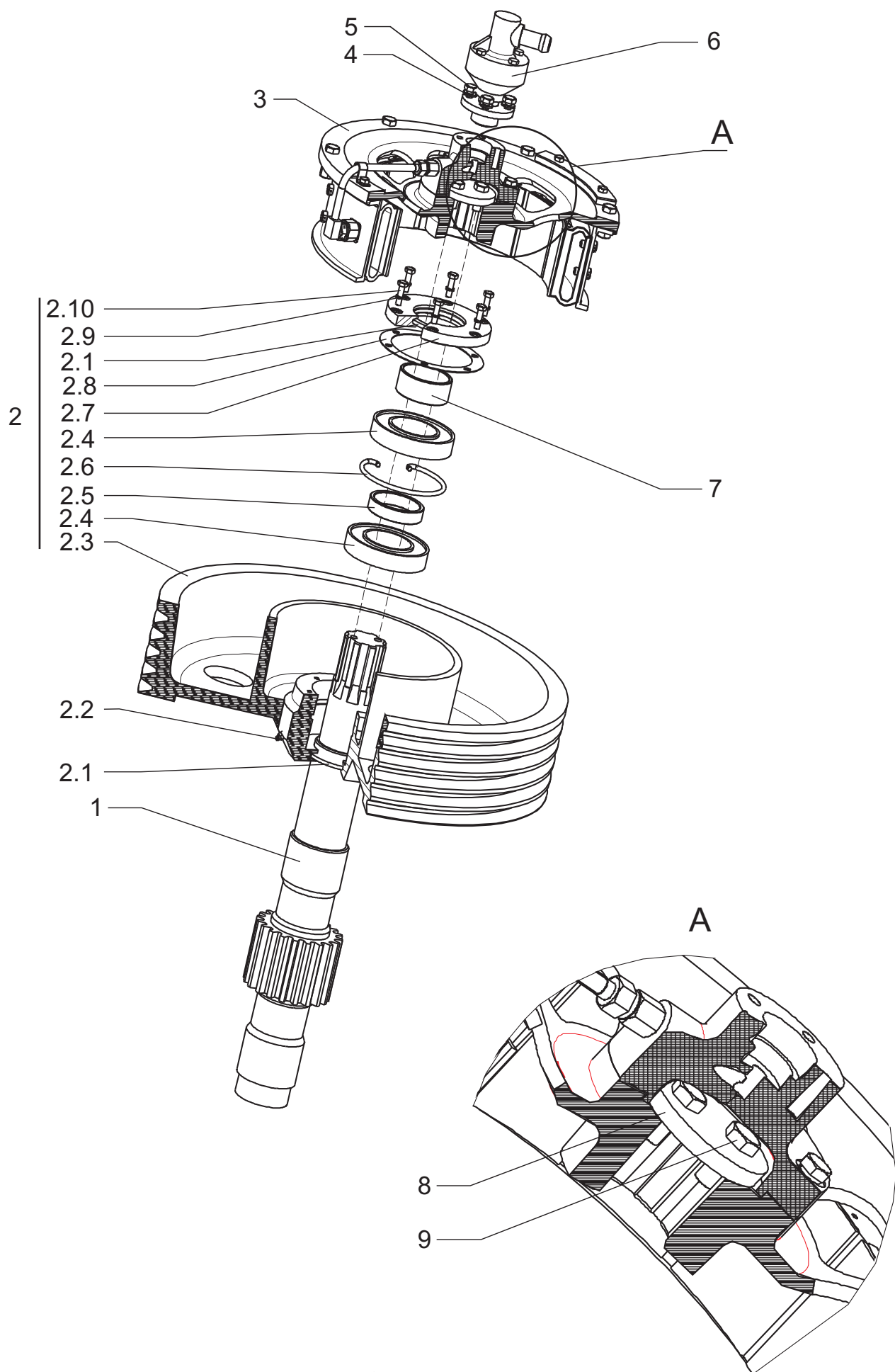
Рисунок 15 - Узел трансмиссионный 03
