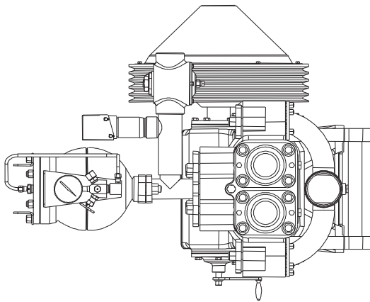
Исполнение 11 (12) - с фрикционной муфтой и шкивом с правой (левой) стороны и боковым расположением манометра
