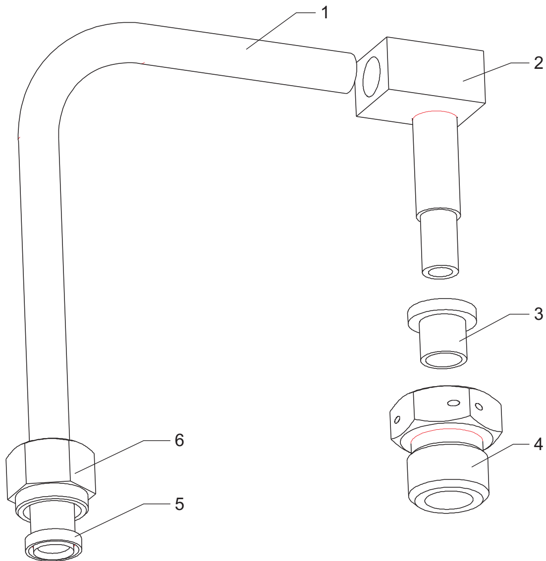
Рисунок 17 - Воздухопровод НБ40.04.110
