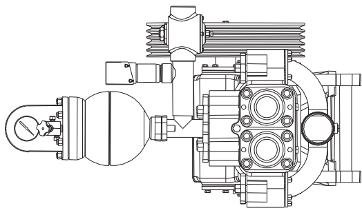
Исполнение 01 (02) - со шкивом с правой (левой) стороны
