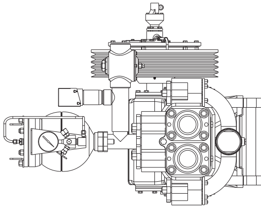
Исполнение 09 (10) - с пневмомуфтой и шкивом с правой (левой) стороны и боковым расположением манометра
