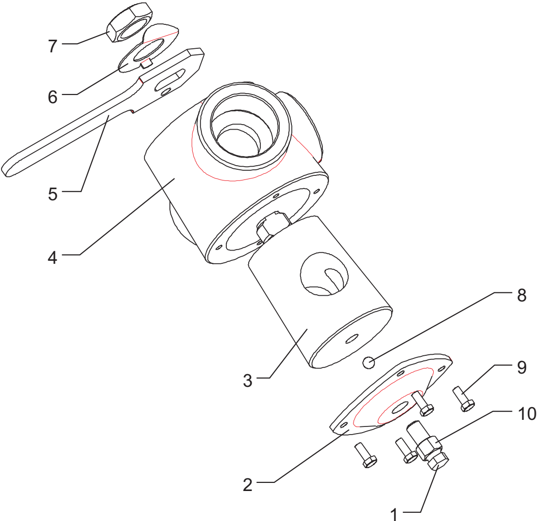
Рисунок 12 - Кран трехходовый НБ40.01.110
