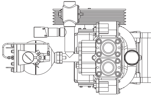
Исполнение 07 (08) - со шкивом с правой (левой) стороны и боковым расположением манометра
